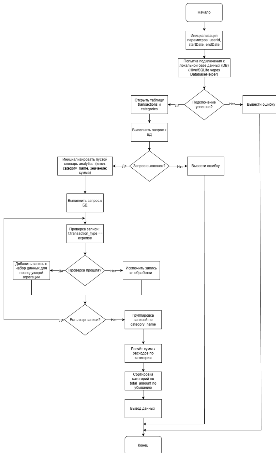
Рисунок 3.3 – Алгоритм агрегации по категориям
